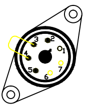
ABS ISO7638 电源线接线定义 (从进线端看插座尾部插孔旁边的编号):
